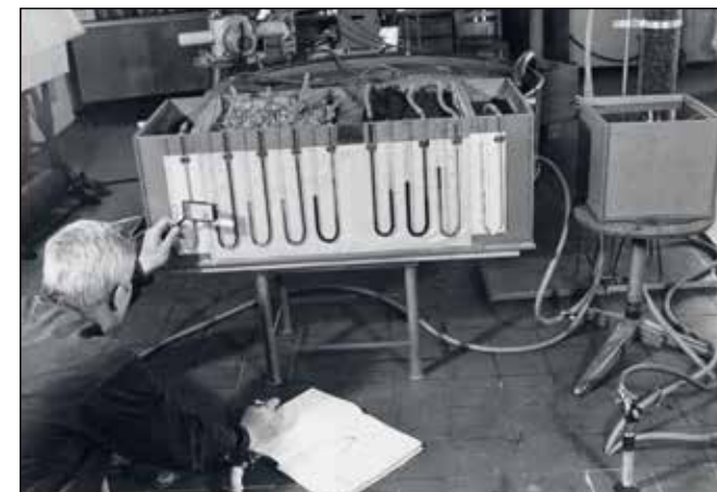
Modelový výzkum migrace jemných částic měřením změn hydraulického spádu, na snímku Jan Skalička, bez datace, foto Renáta Louvarová (Záběhlická) ÚSMH AV ČR, sbírka fotografií
