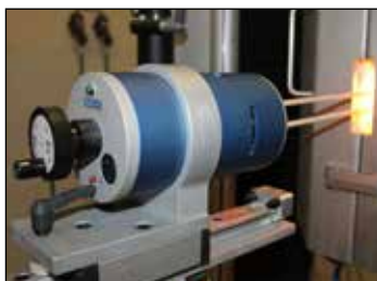
Zařízení Inspekt 100 (Hegewald & Peschke) umožňuje mechanické zkoušky materiálů při vysokých teplotách. Foto: Vlasta Mádllová
