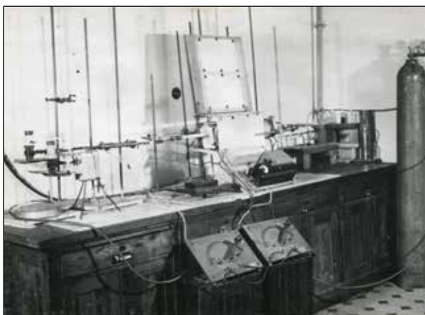
Aparatura pro stanovení kyslíku. Fotografie z výroční zprávy ústavu za rok 1952 NA, fond MPE, k. 110, inv. č. 84
