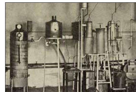
Celkový pohled na karbonizační zařízení. Bylo určeno zejména pro zpracování hnědého uhlí, ale bylo možné v něm karbonizovat i černé spékavé uhlí. In: Zprávy Ústavu pro vědecký výzkum uhlí v Praze , sv. 3, 1937
