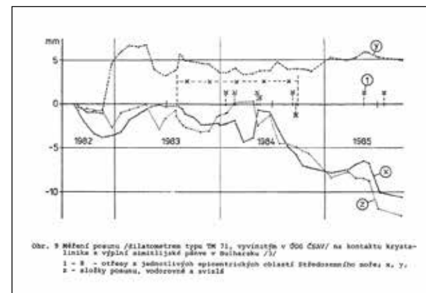
Měření posunu dilatometrem typu TM 71 vyvinutým v Ústavu geologie a geotechniky ČSAV na kontaktu krystalinika s výplní similitijské pánve v Bulharsku /3/ Acta Montana, roč. 78 (1988), s. 21
